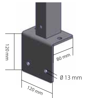
Winkelplatte für Pfosten 60 x 40 mm, angeschweißt
